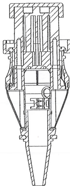
SECTION A-A
