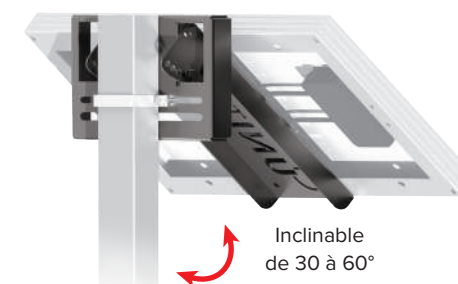
UNIFIX 20S pour Unisun 10.12M/10.24M/20.12M/20.24M Orientation paysage Tête et milieu de mât Ref 0286
