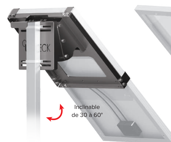
UNIFIX 100S pour Unisun 80.12M/100.12M/110.12BC Orientation paysage ou portrait Tête et milieu de mât Ref 0323
