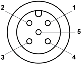
Micro-C M12 5 broches Mâle, vue du câble
